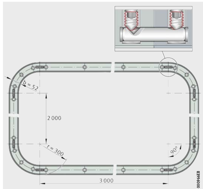
Figure 6 Ovale fermé avec angles de 90° et éléments de liaison des rails VBS LFS52×2000×3000-OV-300-VBS
