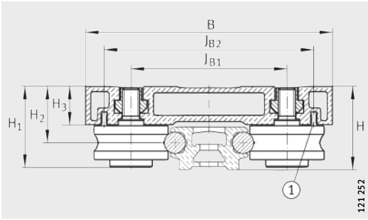
LFCL avec LFS (-C, -CE, -CEE, -E, -EE, -N, -NZZ)
