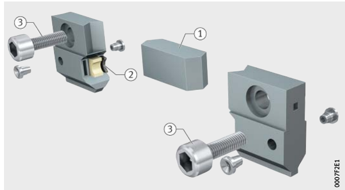
Figure 1 Racleurs-graisseurs AB
