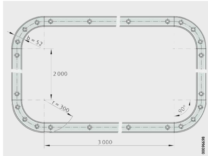
Figure 5 Ovale fermé avec angle à 90° LFS52×2000×3000-OV-300
