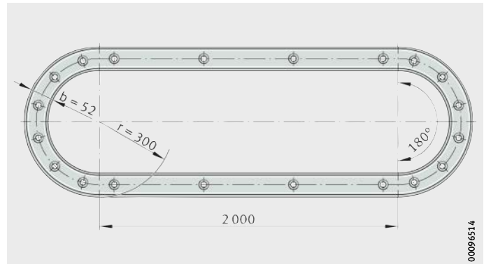
Figure 3 Ovale fermé avec angle à 180^\circ LFS52×2000-OV-300
