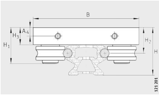
LFL-SF avec LFS (-C, -CE, -CEE, -E, -EE, -NZZ)
