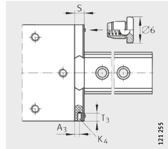
AB Vue tournée de 90°
