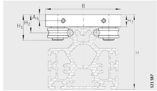
LFL avec LFS..-M 3 )
