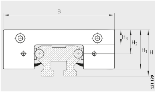
LFKL-SF avec LFS (-C, -CE, -CEE, -E, -EE, -NZZ)
