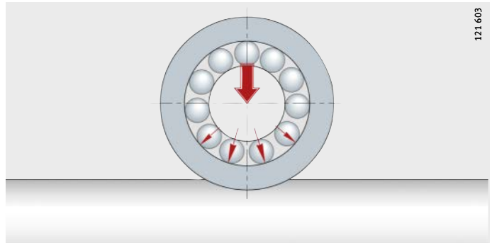
Figure 1 Déformation de la bague extérieure en cas d'appui sur un chemin de roulement
