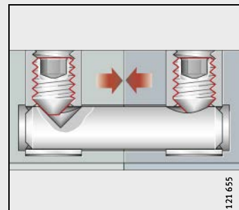
Eléments de liaison pour rails VBS
