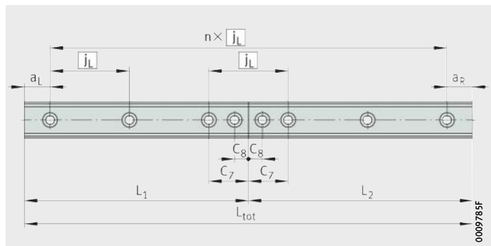
Figure 4 Trou supplémentaire
