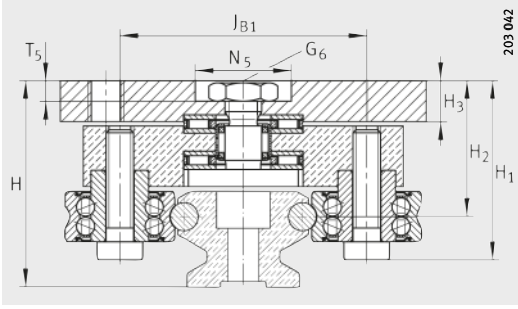
LFDL-SF avec LFS (-C, -CE, -CEE, -E, -EE, -NZZ)
