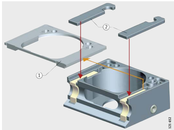
Figure 2 Montage sur le chariot LFCL
