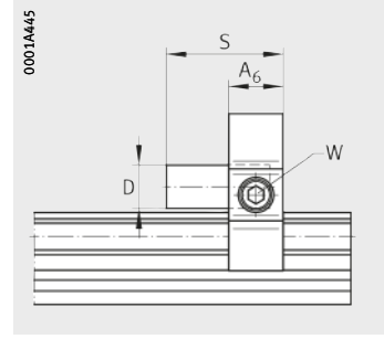
PAH Vue tournée de 90°
