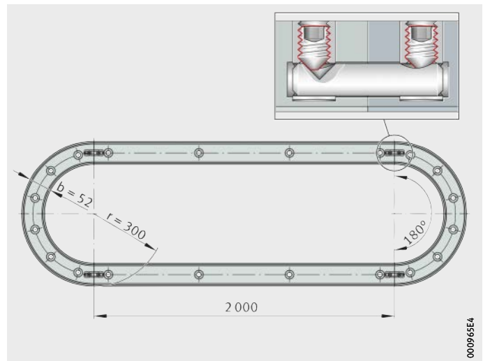
Figure 4 Ovale fermé avec angles de 180^\circ et éléments de liaison des rails VBS LFS52×2000-OV-300-VBS
