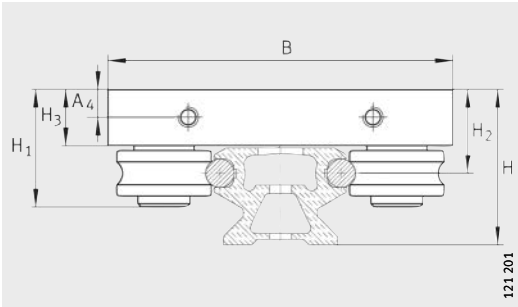
LFL avec LFS (-C, -CE, -CEE, -E, -EE, -NZZ)
