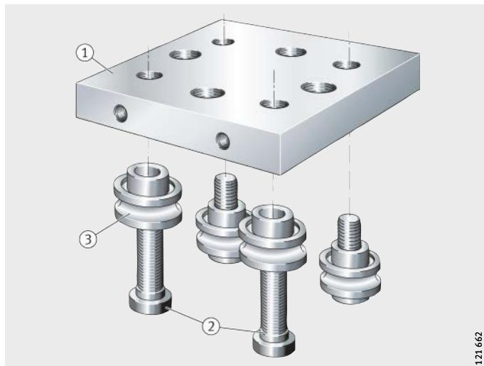
Figure 3 Chariot ouvert
